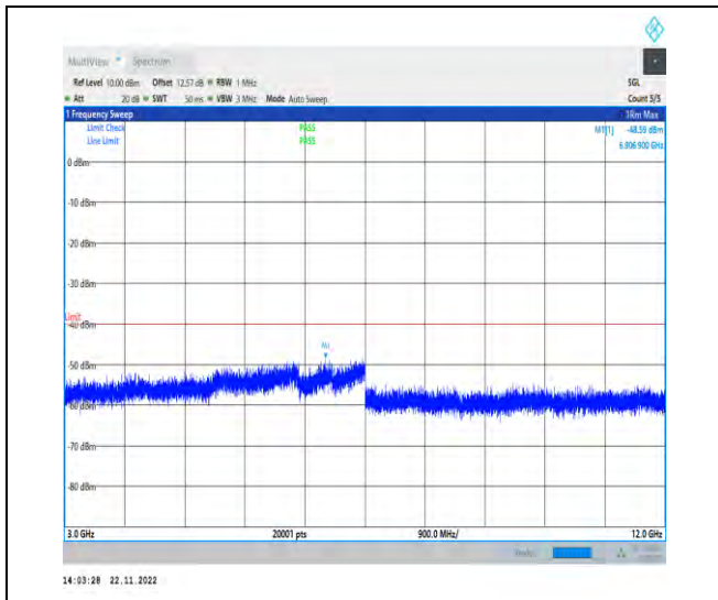
1-N30-PC3-15-10-M-1-DFT-PI2BPSK-Inner_1RB_L eft-1@1-3000-12000-Ant1-6906.90--48.59--40-PAS
