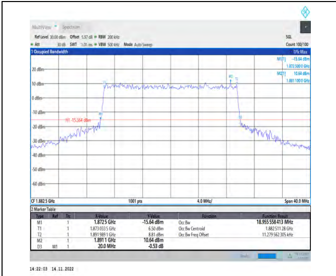
1-N25-PC3-15-20-M-7-CP-16QAM-Outer_Full-106@ 0-Ant1-18.956-20.000-≤20-PASS
