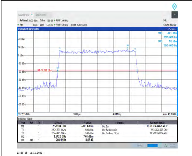
1-N7-PC3-15-20-M-9-CP-256QAM-Outer_Full-106@0 0-Ant1-18.913-20.000-≤20-PASS
