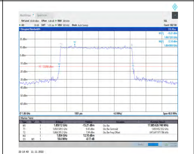
1-N2-PC3-15-20-L-3-DFT-16QAM-Outer_Full-100@ 0-Ant1-17.886-18.600-≤20-PASS
