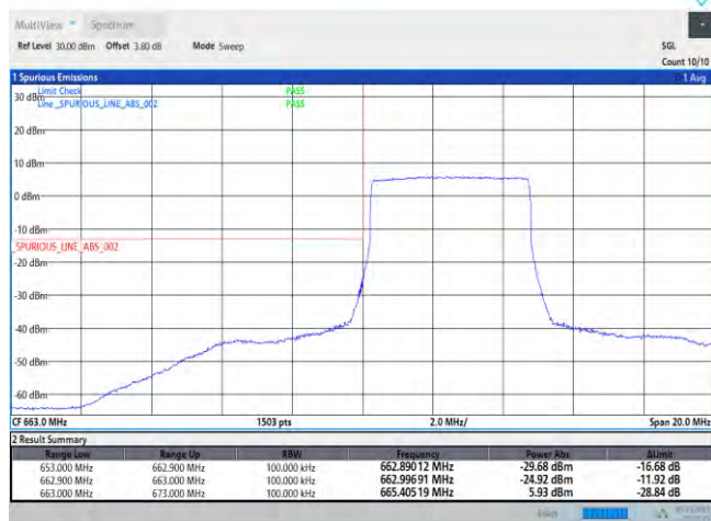
Band71-5MHz-QPSK-133147-25RB#0
