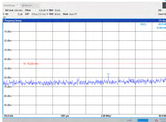
Band41-20MHz-QPSK-39750-1RB#0-Range2:0.15~30MHz
