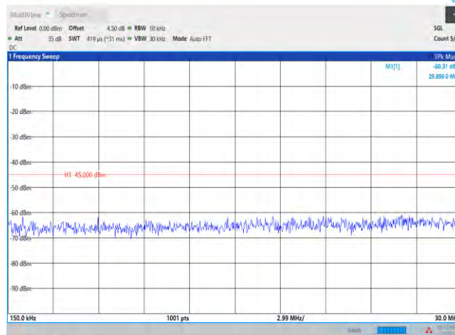
Band7-20MHz-QPSK-20850-1RB#0-Range2:0.15~30MHz
