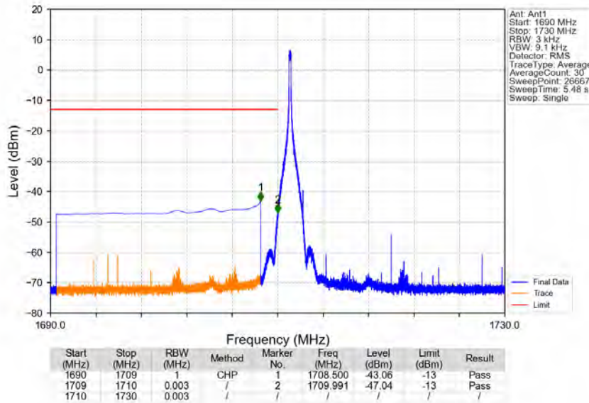
Band66_20MHz_16QAM_LCH_1720MHz_RB_1_0_NTNV
