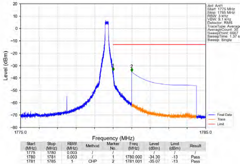
Band66_5MHz_QPSK_HCH_1777.5MHz_RB_1_24_NTNV
