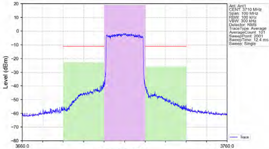
Band43d 20MHz 64QAM LCH 3710MHz RB 100 0 NTN
