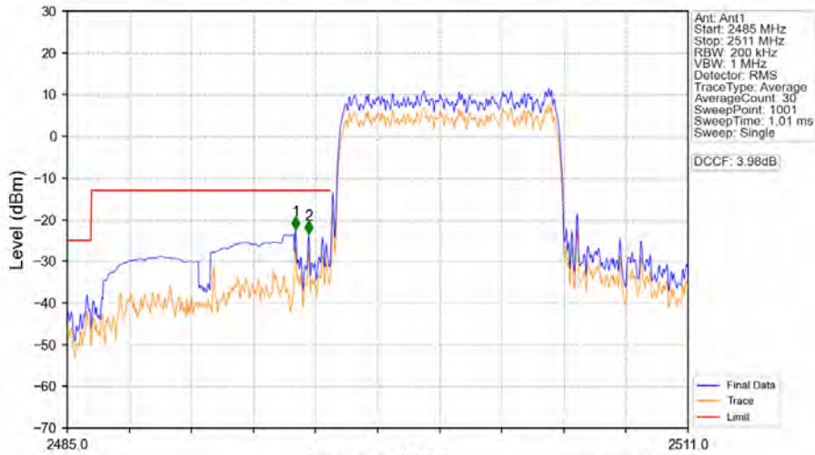
Band41_10MHz_QPSK_LCH_2501MHz_RB_50_0_NTNV
