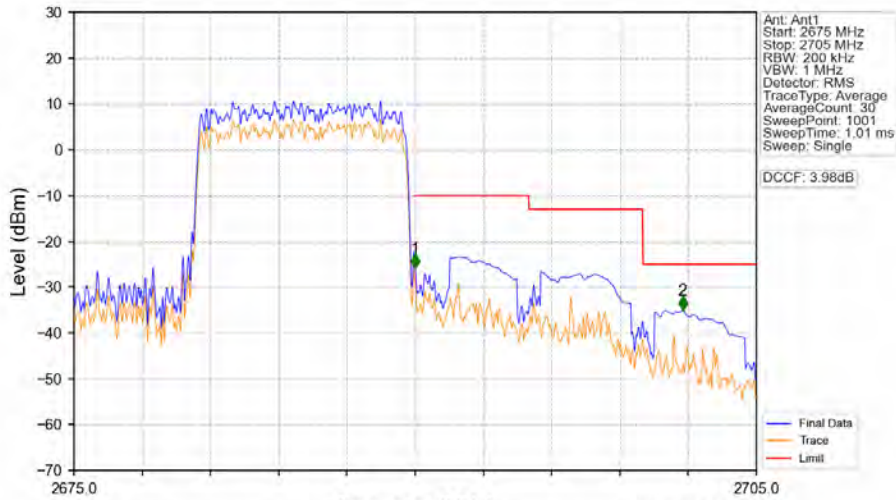
Band41_10MHz_QPSK_HCH_2685MHz_RB_50_0_NTNV
