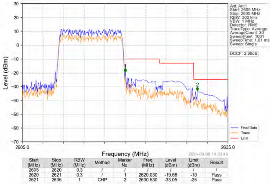
Band38_10MHz_QPSK_HCH_2615MHz_RB_50_0_NTNV
