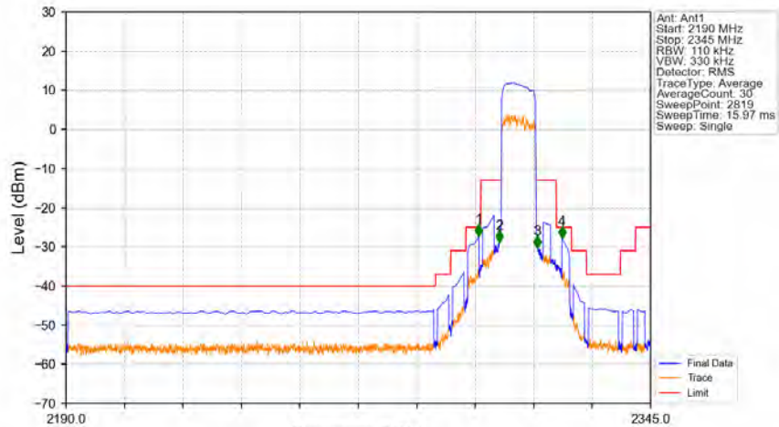
Band30_10MHz_QPSK_MCH_2310MHz_RB_50_0_NTNV
