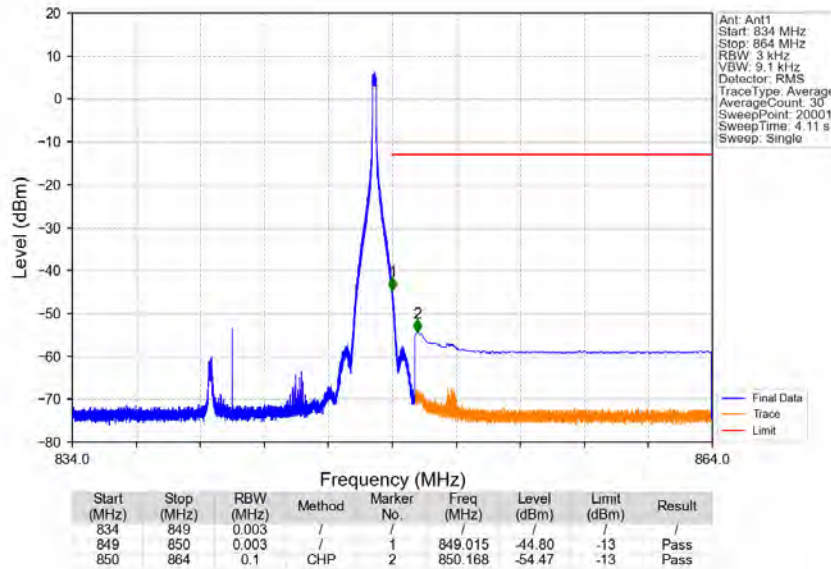
Band26c_15MHz_16QAM_HCH_841.5MHz_RB_1_74_NTNV
