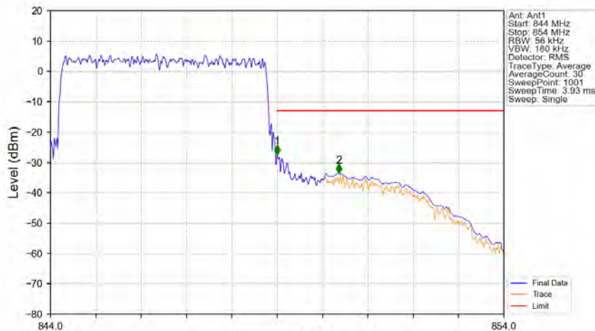
Band26b 5MHz QPSK HCH 846.5MHz RB 25 0 NTV
