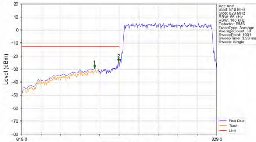
Band26b 5MHz QPSK LCH 826.5MHz RB 25 0 NTV
