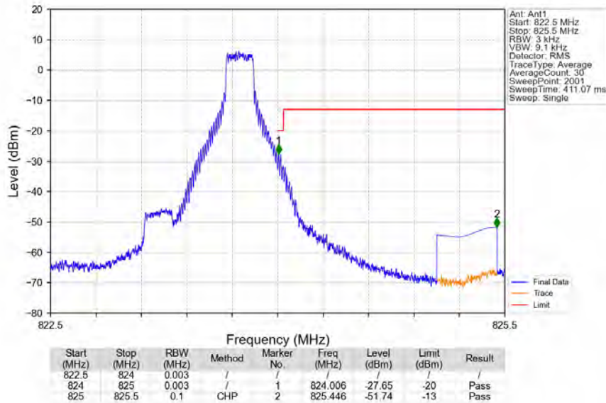
Band26a 1.4MHz 16QAM HCH 823.3MHz_RB 1 5 NTV
