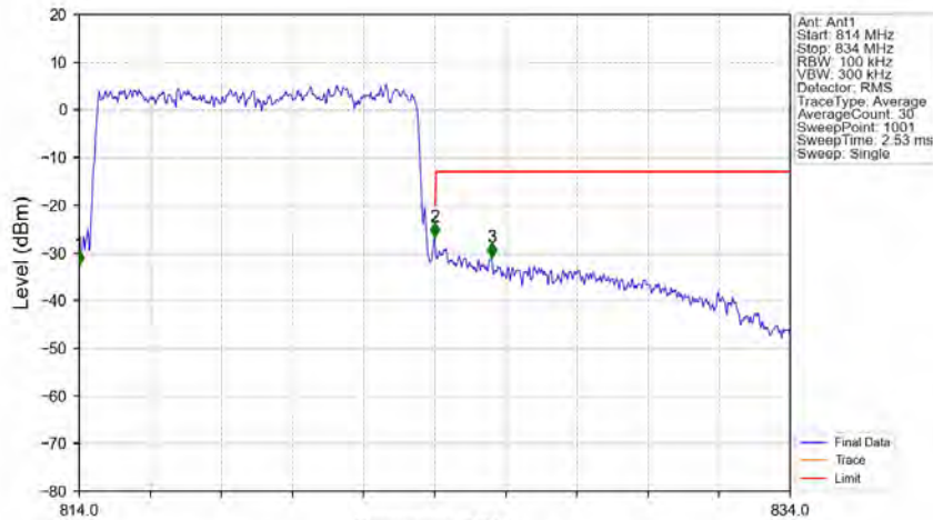
Band26a_10MHz_QPSK_MCH_819MHz_RB_50_0_NTNV
