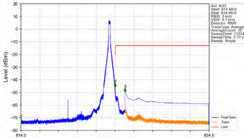
Band26a 10MHz QPSK HCH 819MHz RB 1 49 NTN
