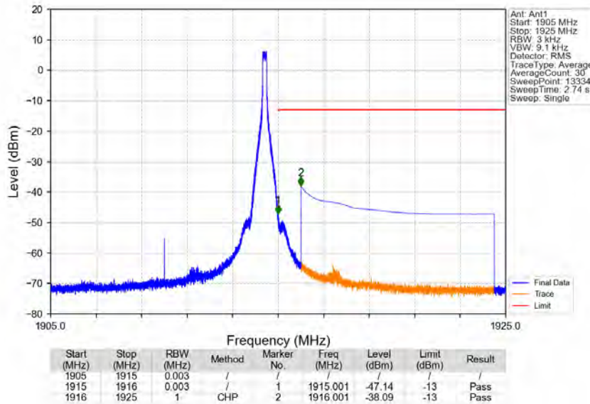
Band25_10MHz_QPSK_HCH_1910MHz_RB_1_49_NTNV
