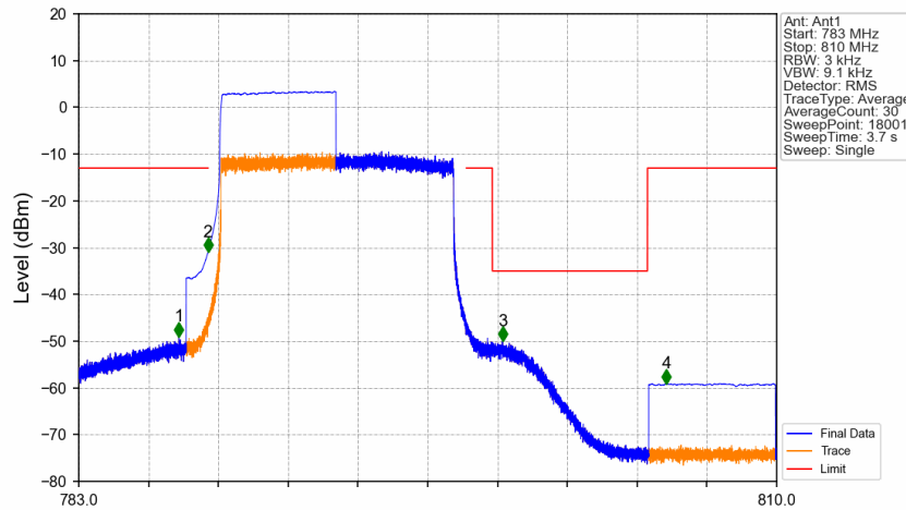
Band14_10MHz_QPSK_MCH_793MHz_RB_50_0_NTNV
