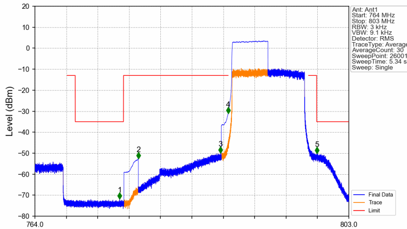
Band14_10MHz_QPSK_LCH_793MHz_RB_50_0_NTNV
