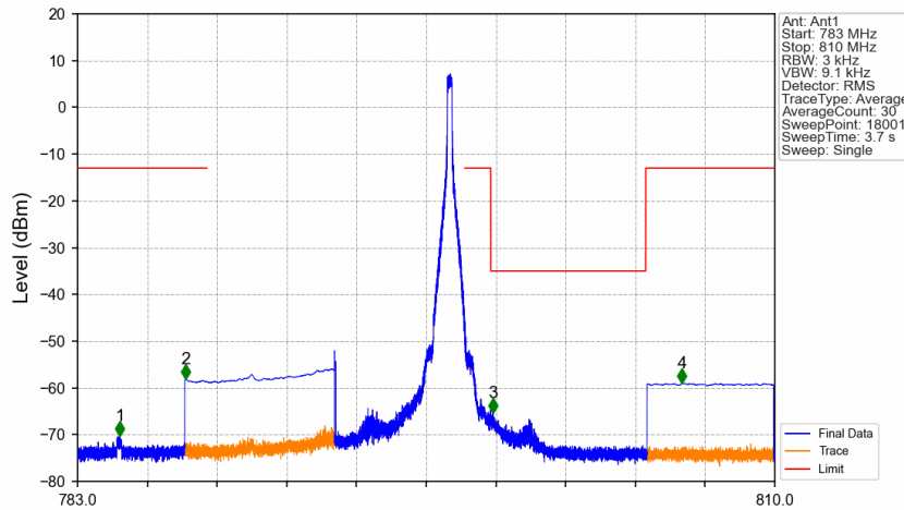
Band14_10MHz_QPSK_HCH_793MHz_RB_1_49_NTNV
