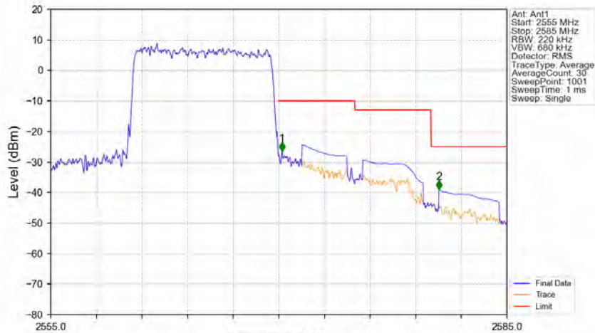
Band7_10MHz_QPSK_HCH_2565MHz_RB_50_0_NTNV
