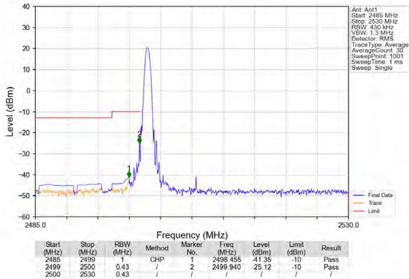
Band7_20MHz_64QAM_LCH_2510MHz_RB_1_0_NTNV
