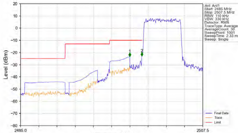
Band7_5MHz_QPSK_LCH_2502.5MHz_RB_25_0_NTNV
