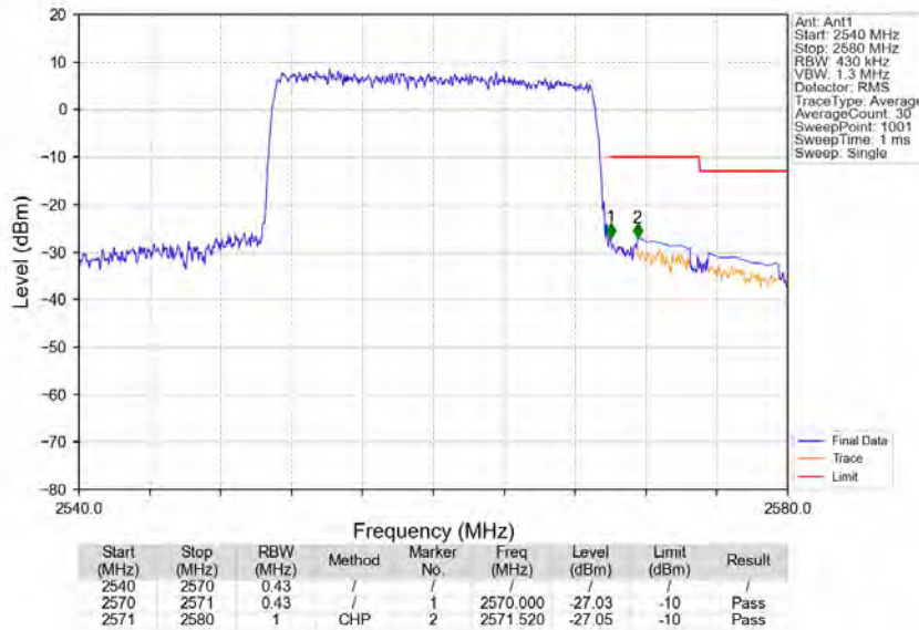
Band7_20MHz_QPSK_HCH_2560MHz_RB_100_0_NTNV
