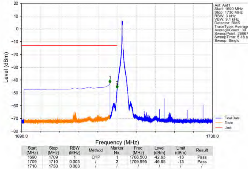
Band4_20MHz_16QAM_LCH_1720MHz_RB_1_0_NTNV
