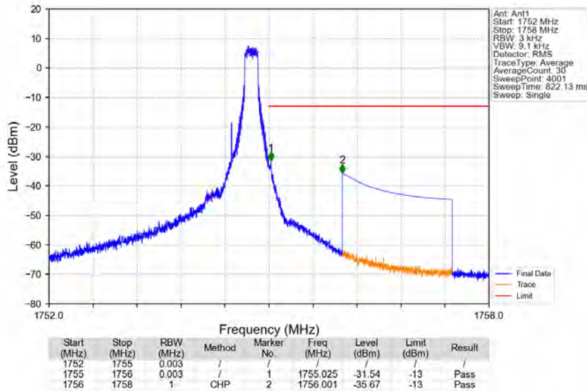
Band4_3MHz_QPSK_HCH_1753.5MHz_RB_1_14_NTNV
