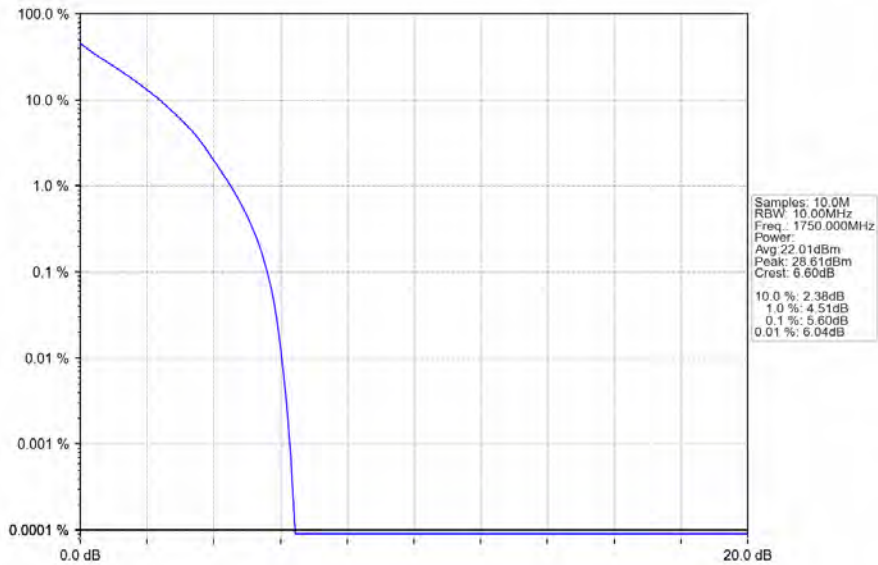
Band4_10MHz_QPSK_HCH_1750MHz_RB_50_0_NTNV
