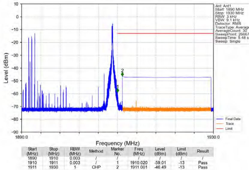
Band2_20MHz_64QAM_HCH_1900MHz_RB_1_99_NTNV
