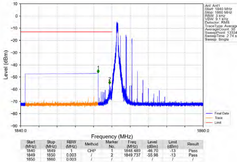
Band2_10MHz_64QAM_LCH_1855MHz_RB_1_0_NTNV
