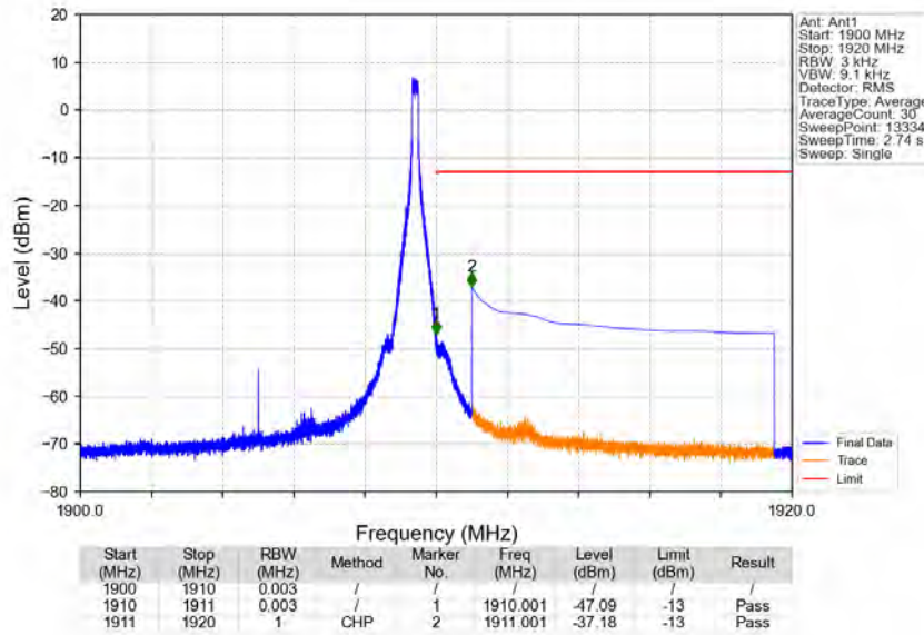
Band2_10MHz_QPSK_HCH_1905MHz_RB_1_49_NTNV
