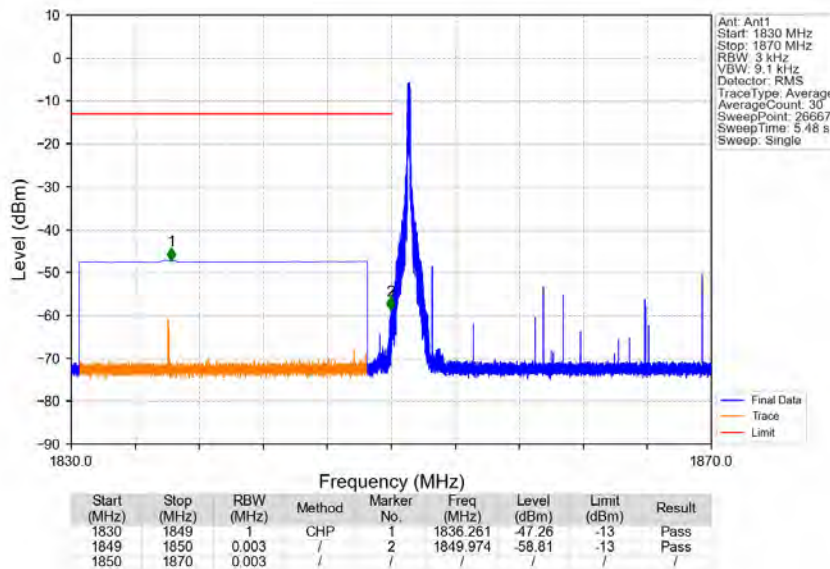
Band2_20MHz_64QAM_LCH_1860MHz_RB_1_0_NTNV
