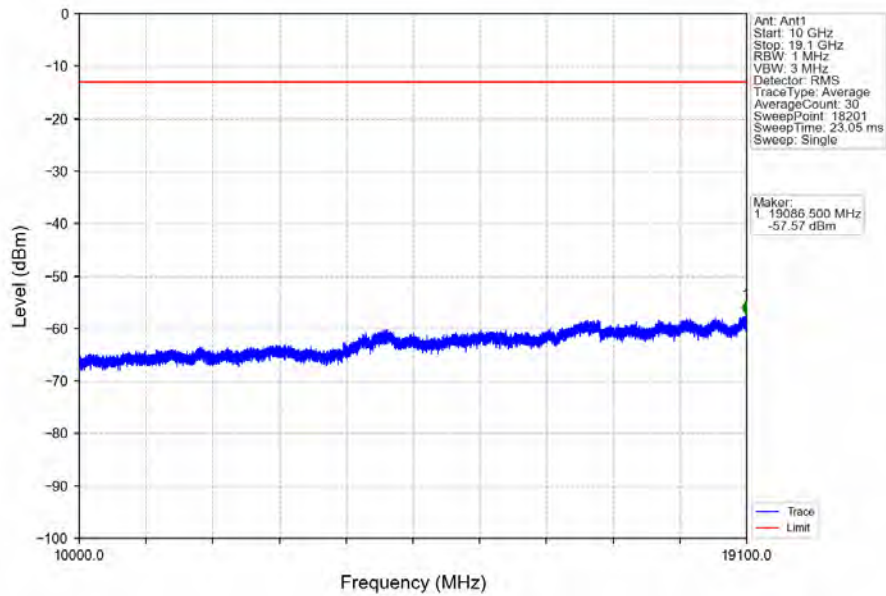
Band2_20MHz_16QAM_LCH_1860MHz_RB_100_0_NTNV
