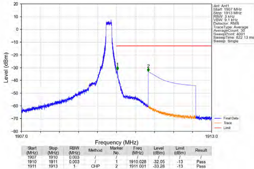
Band2_3MHz_QPSK_HCH_1908.5MHz_RB_1_14_NTNV
