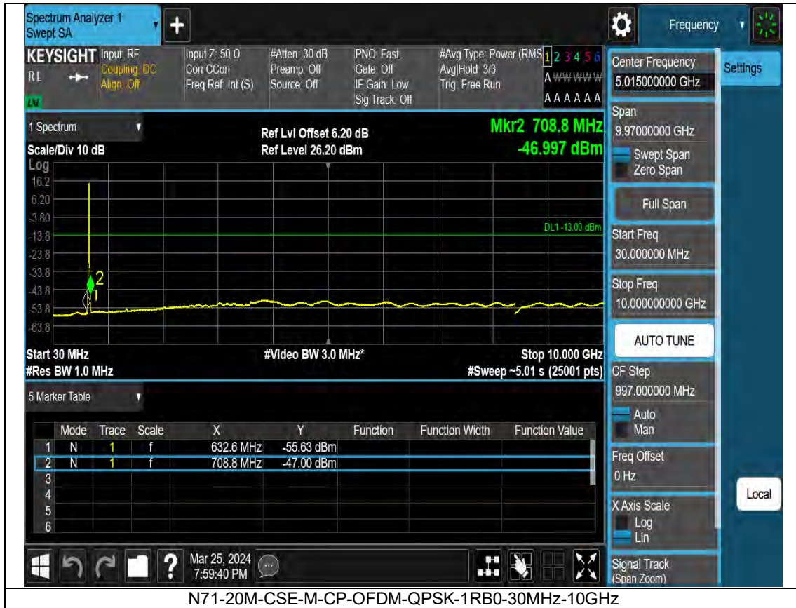
N71-20M-CSE-M-CP-OFDM-QPSK-1RB0-30MHz-10GHz
