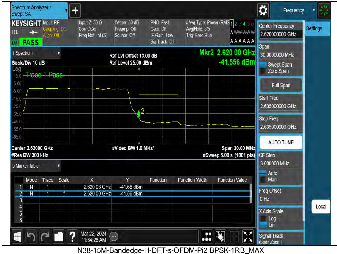
N38-15M-Bandedge-H-DFT-s-OFDM-Pi2 BPSK-1RB_MAX
