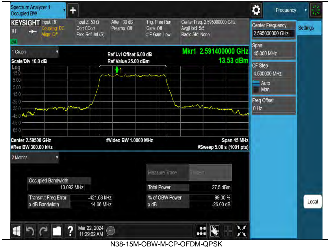
N38-15M-OBW-M-CP-OFDM-QPSK
