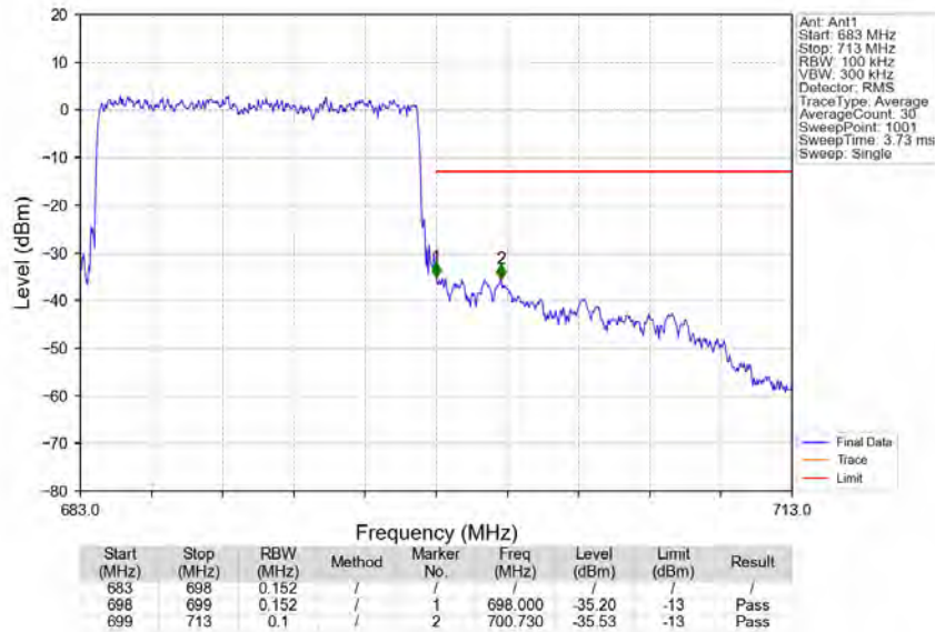
Band71 15MHz QPSK HCH 690.5MHz RB 75 0 NTV
