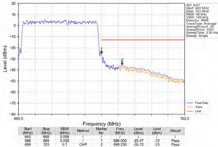
Band71 5MHz QPSK HCH 695.5MHz RB 25 0 NTV
