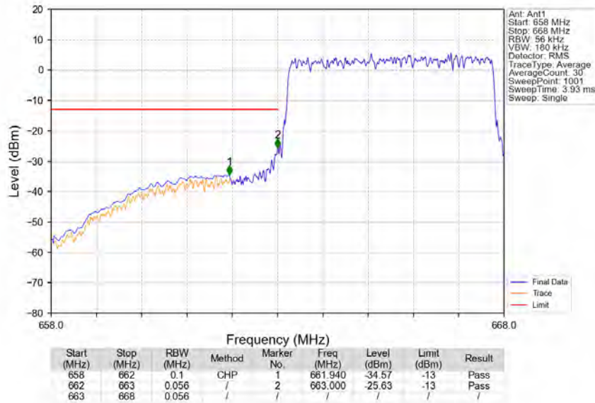
Band71_5MHz_QPSK_LCH_665.5MHz_RB_25_0_NTNV
