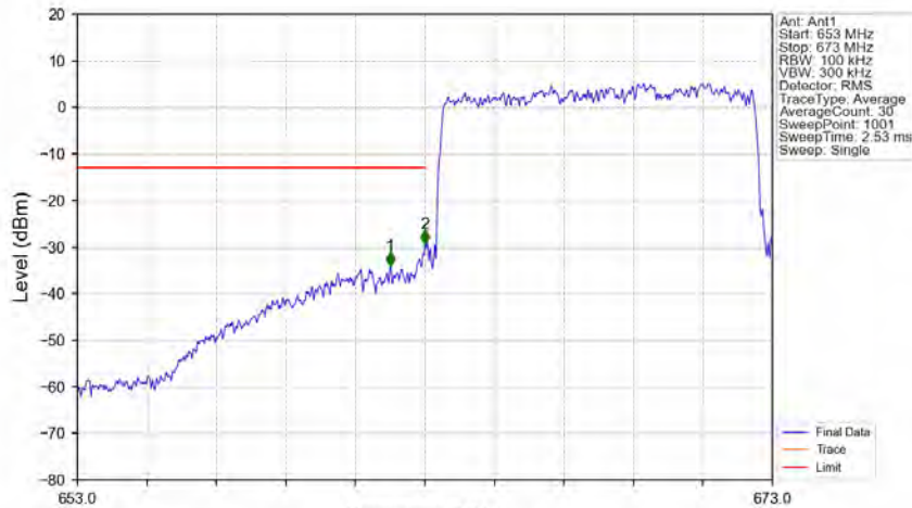
Band71_10MHz_QPSK_LCH_668MHz_RB_50_0_NTNV
