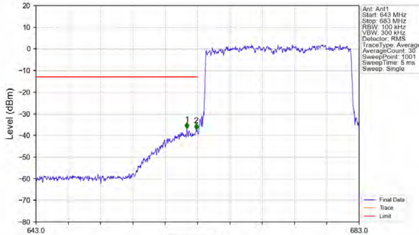
Band71_20MHz_QPSK_LCH_673MHz_RB_100_0_NTNV
