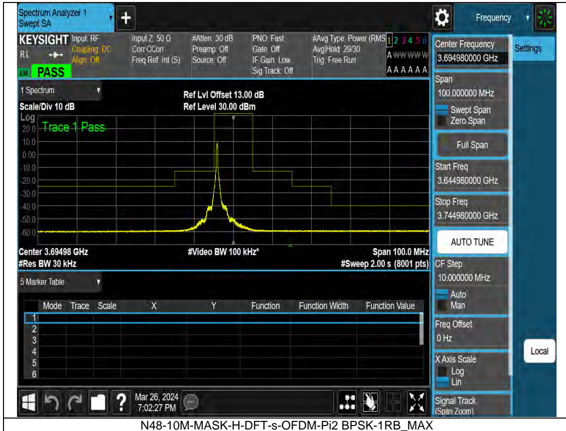
N48-10M-MASK-H-DFT-s-OFDM-Pi2 BPSK-1RB_MAX
