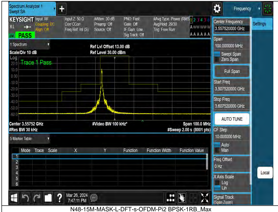
N48-15M-MASK-L-DFT-s-OFDM-Pi2 BPSK-1RB_Max
