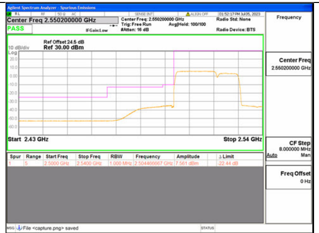
7C / 20+10MHz / Low CH / QPSK / 100#0-50#0
