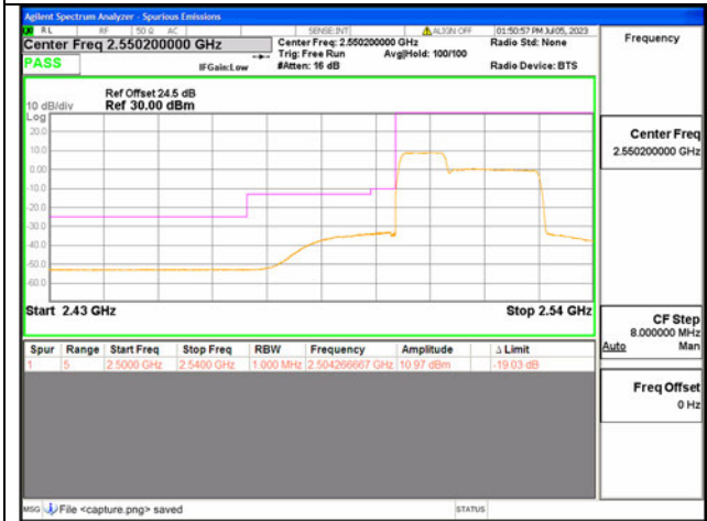
7C / 10+20MHz / Low CH / QPSK / 50#0-100#0
