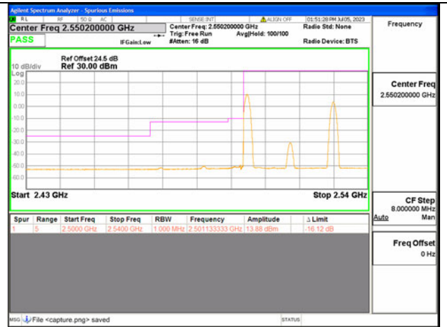
7C / 20+10MHz / Low CH / QPSK / 1#0-1#49
