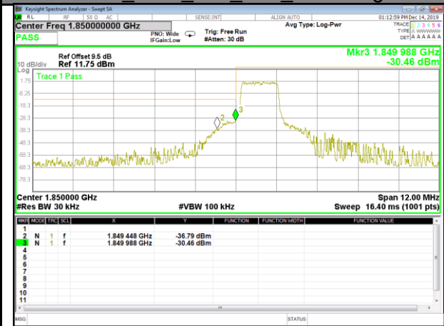
QPSK 1.4M 6#0 Low Band edge
