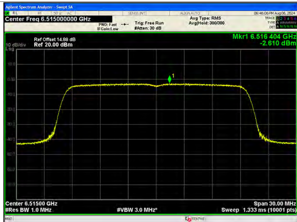
PSD NVNT ax20 6515MHz Ant2 SISO
