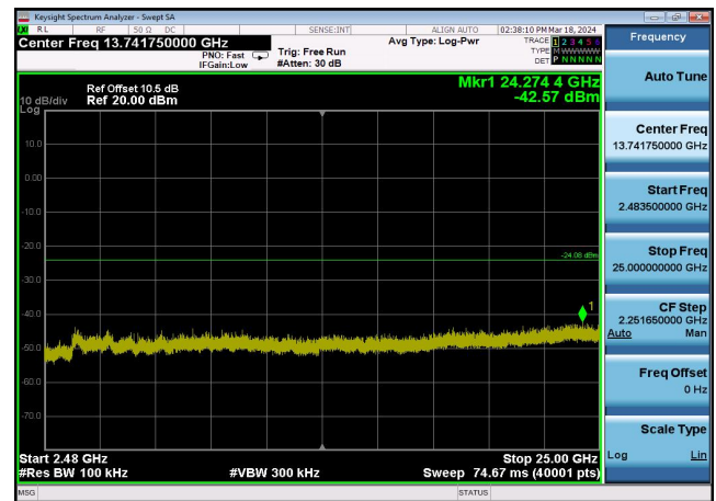
,Plot 4,2483.5MHz~25000MHz-802.11ax(2 0MHz),2462MHz,Ant0
