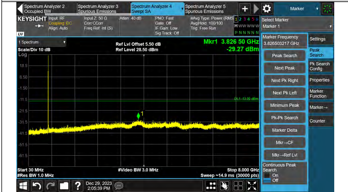
Band12-5MHz-QPSK-23155-1RB#0-30~8000MHz
