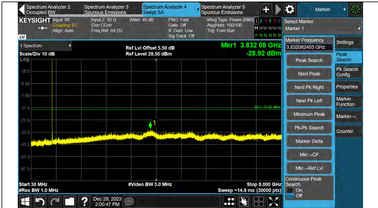
Band12-5MHz-QPSK-23095-1RB#0-30~8000MHz
