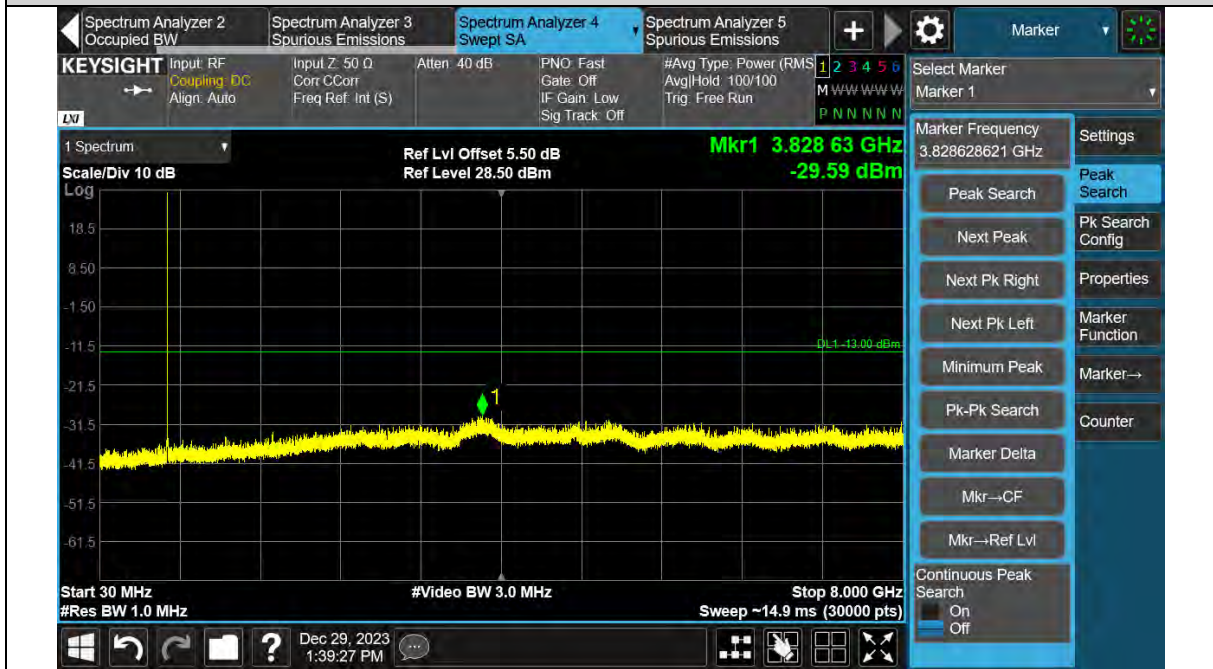
Band12-3MHz-QPSK-23095-1RB#0-30~8000MHz
