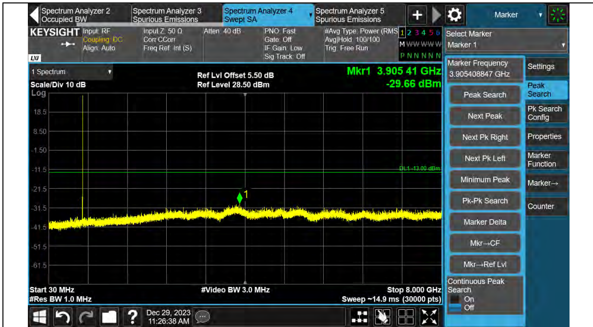
Band12-3MHz-QPSK-23025-1RB#0-30~8000MHz
