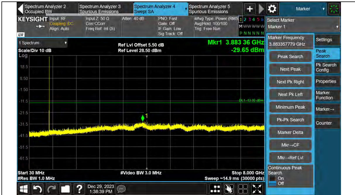
Band12-3MHz-QPSK-23165-1RB#0-30~8000MHz
