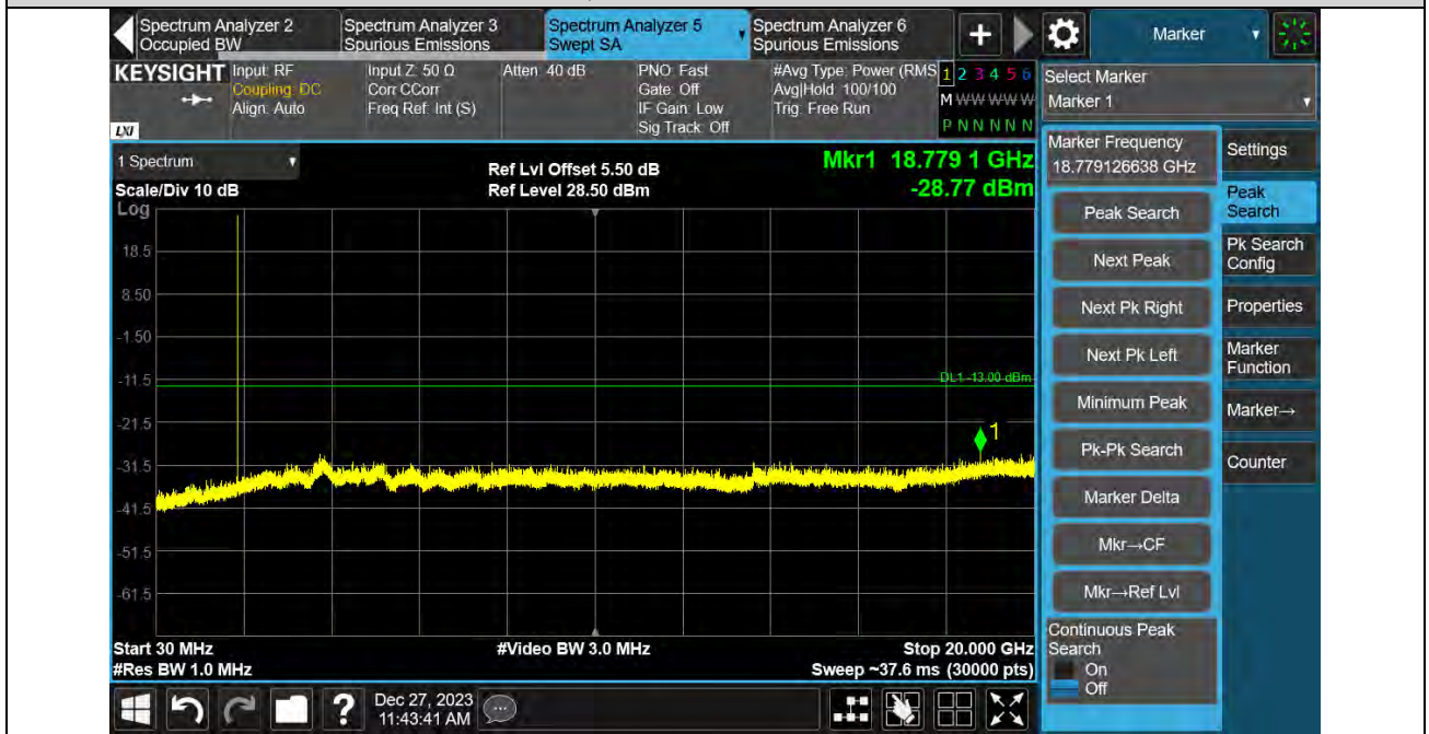
Band2-3MHz-QPSK-19185-1RB#0-30~20000MHz
