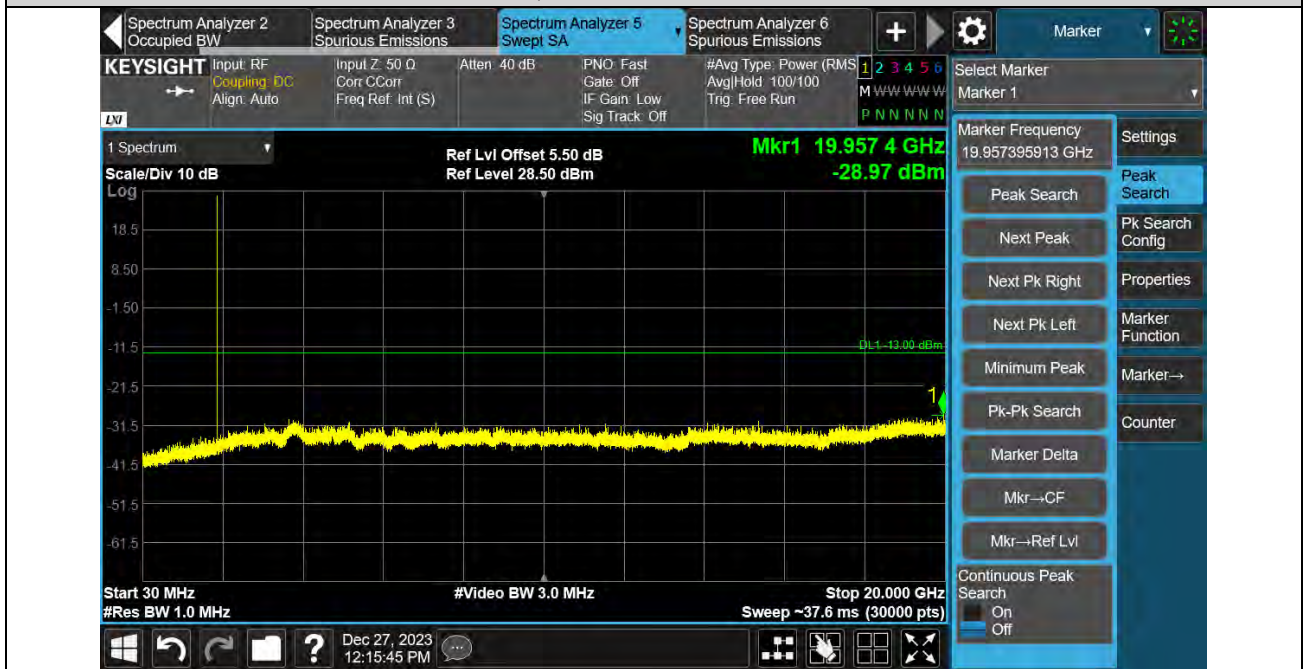
Band2-5MHz-QPSK-19175-1RB#0-30~20000MHz
