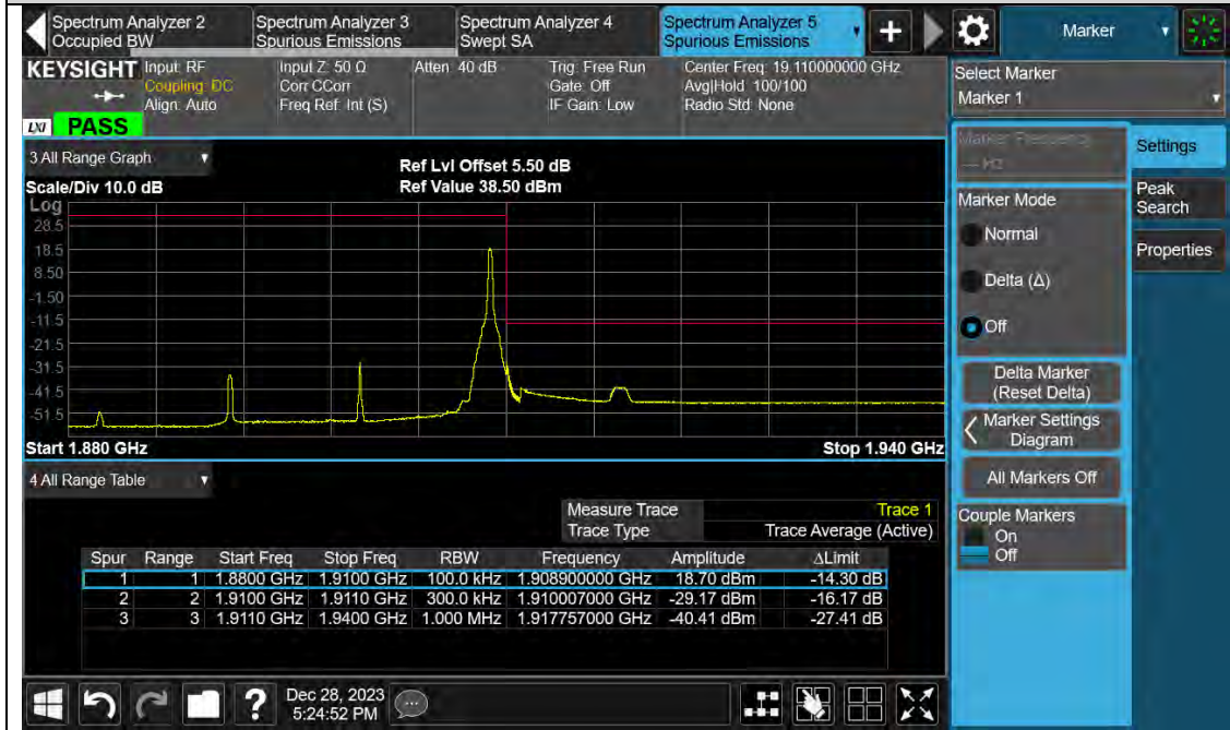
Band2-20MHz-16QAM-19100-100RB#0
