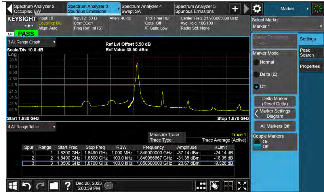
Band2-10MHz-QPSK-18650-50RB#0
