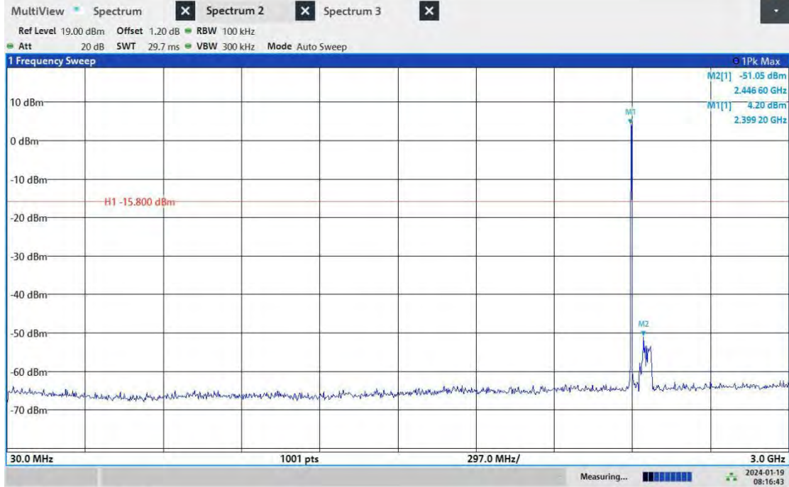
DH5_Ant1_2402_30~3000
