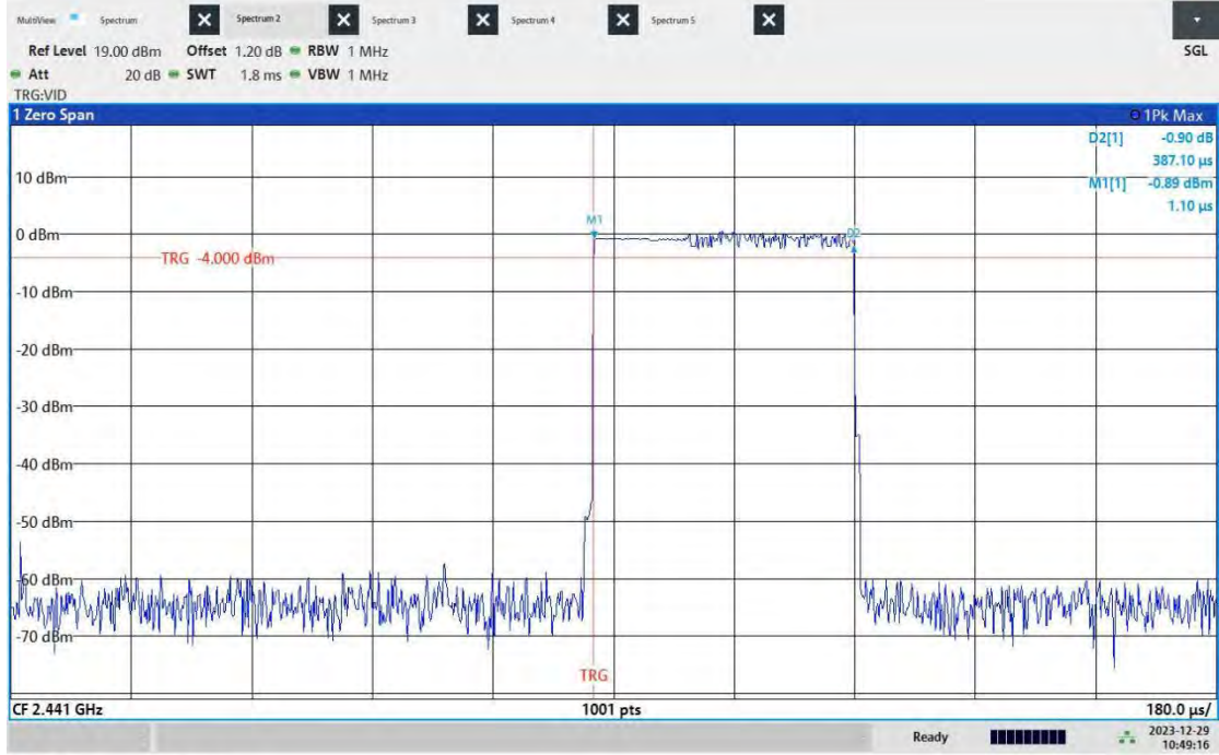
2DH1_Ant1_Hop
