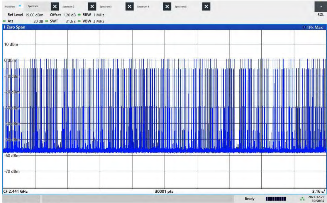
2DH3_Ant1_Hop
