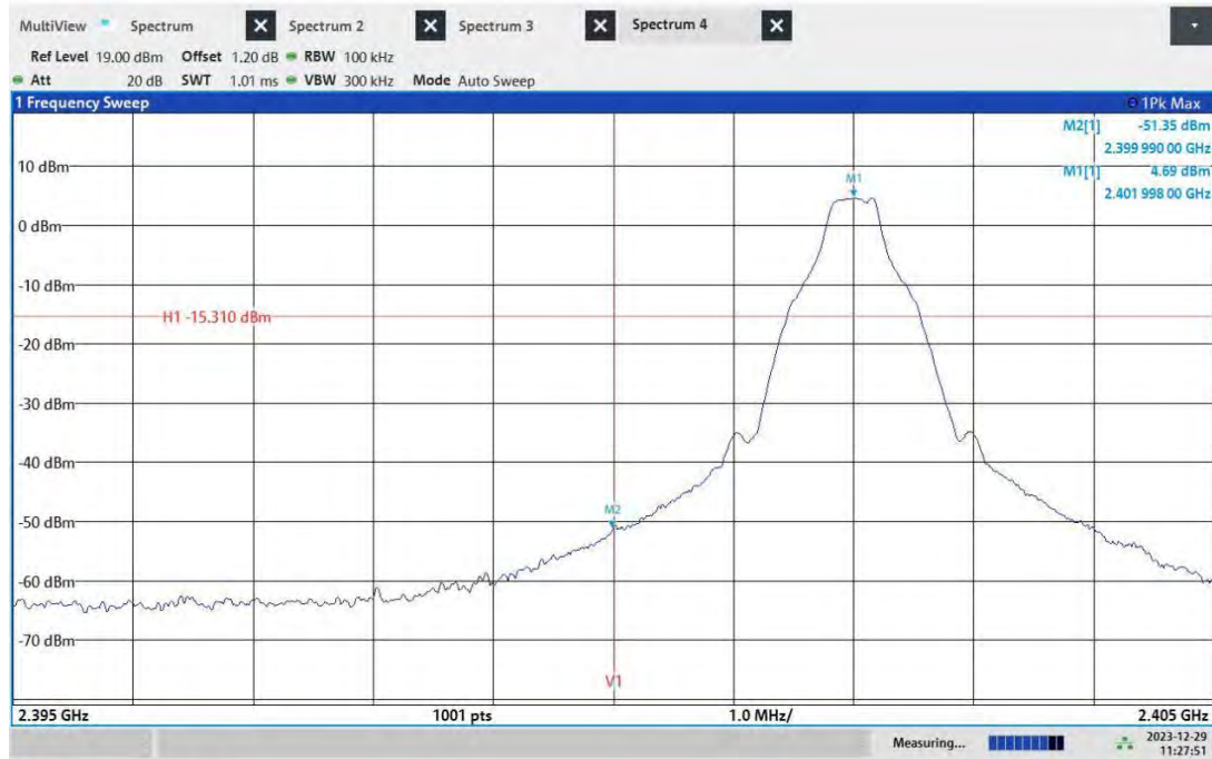
DH5_Ant1_Low_2402
