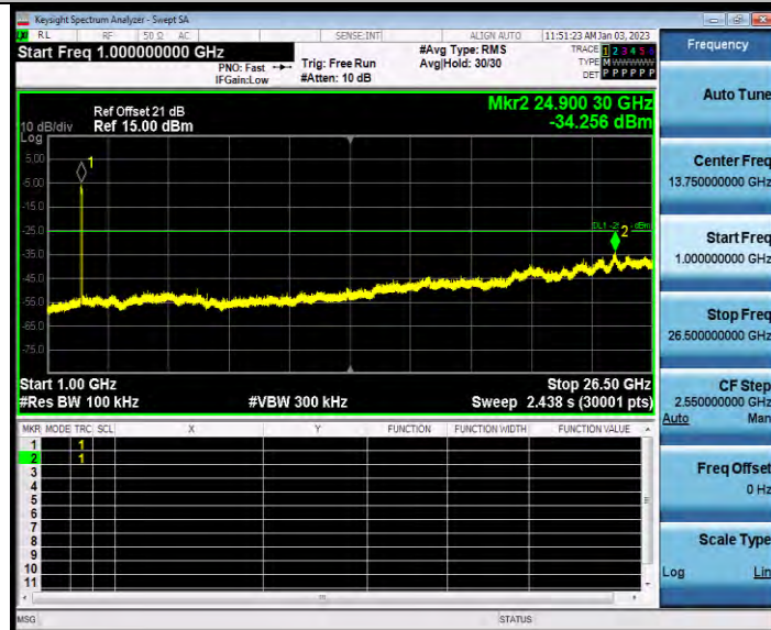
11AX40MIMO_Ant1_2452_0~Reference
