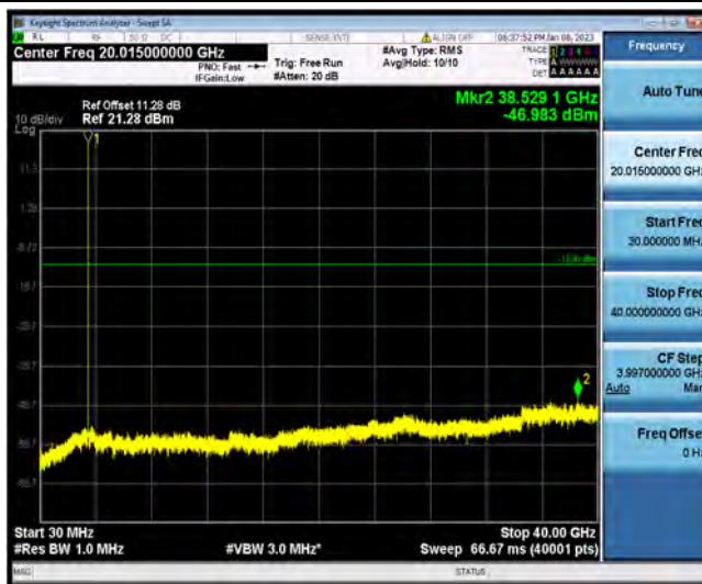
N78-60MHz-QPSK-634666-1RB#0-Range 1:30~40000MHz
