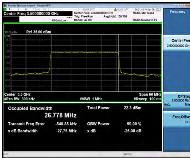
N78-30MHz-256QAM-633334-75RB#0
