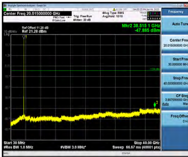
N78-60MHz-QPSK-632000-1RB#0-Range 1:30~40000MHz
