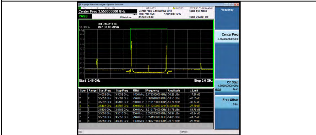
42-42-20MHz-20MHz-64QAM-64QAM-42792-42990-1RB#99-1RB#0
