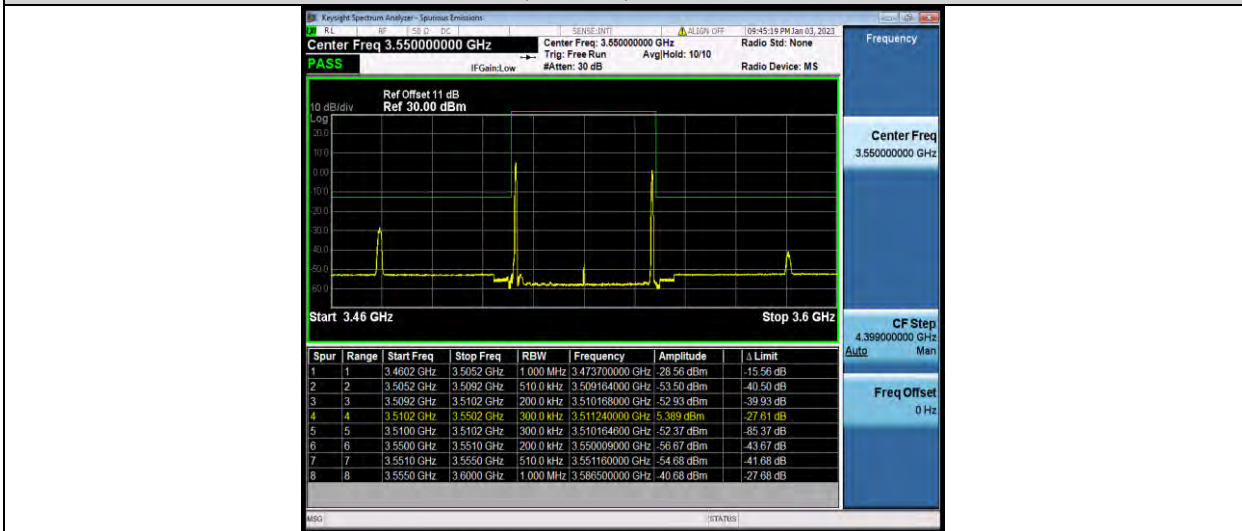
42-42-20MHz-20MHz-16QAM-16QAM-42792-42990-1RB#99-1RB#0
