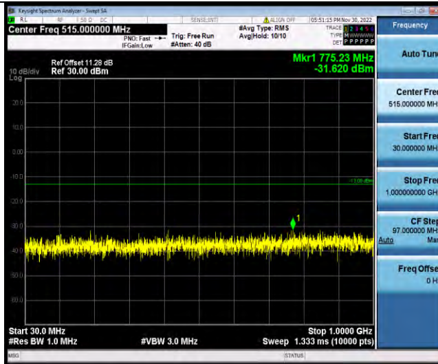
Band25-15MHz-QPSK-26365-1RB#0-Range2:1000~20000MHz
