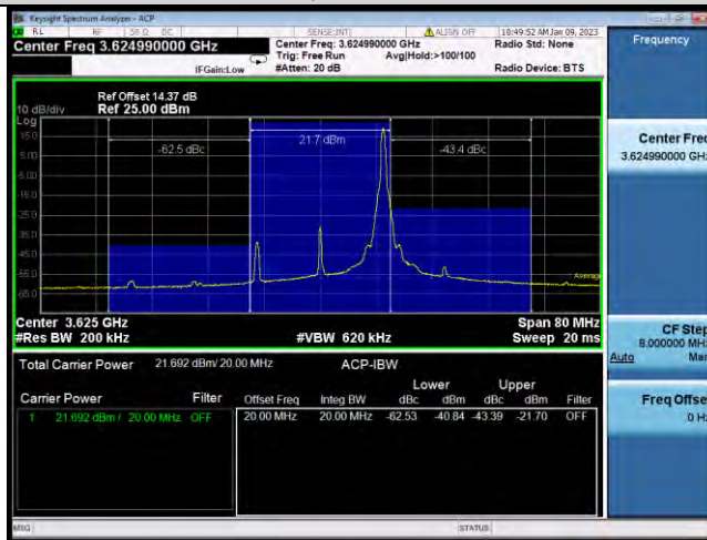
N48-20MHz-QPSK-641666-50RB#0
