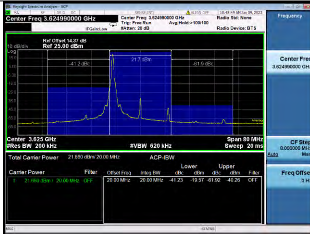
N48-20MHz-QPSK-641666-1RB#50
