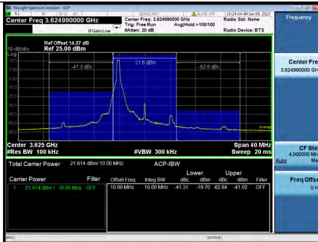
N48-10MHz-QPSK-641666-1RB#24
