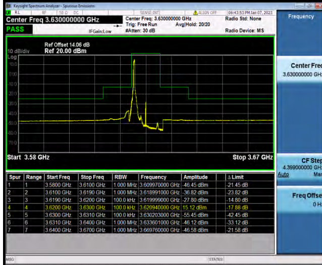
N48-10MHz-QPSK-641666-1RB#24
