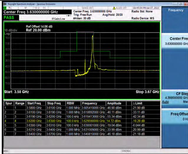
N48-10MHz-QPSK-641666-25RB#0
