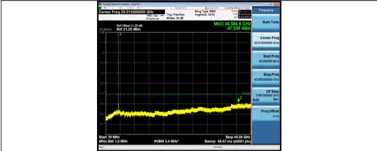
N48-20MHz-QPSK-641666-1RB#0-Range1:30~40000MHz
