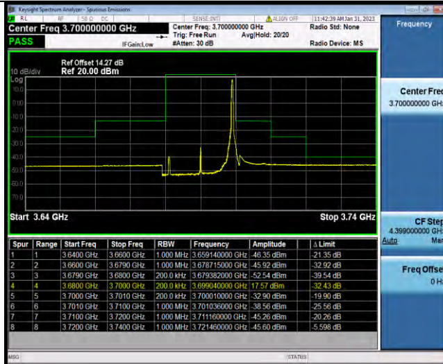
N48-20MHz-QPSK-646000-50RB#0
