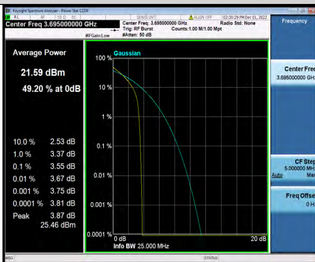
Band48-10MHz-QPSK-56690-50RB#0
