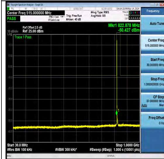
NTNV-N5-PC3-15-10-L-DFT-QPSK-Edge_1RB_L eft-Ant2-PASS
