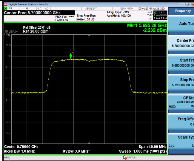
11AX20MIMO Ant9 5700
