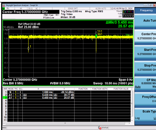
11N40MIMO Ant9 5270
