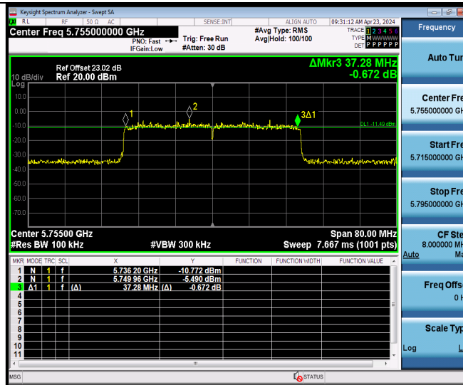
11AX40MIMO Ant9 5755
