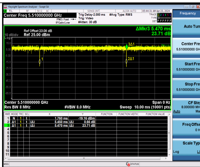
11AX40MIMO Ant9 5510
