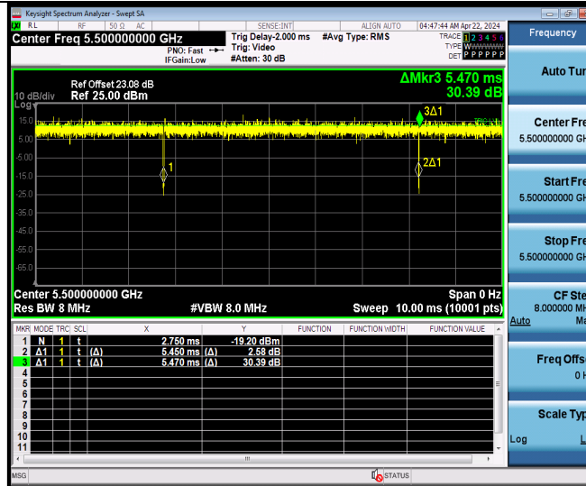
11AX20MIMO Ant9 5500
