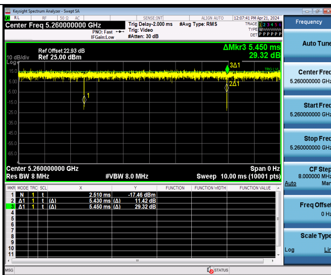
11N20MIMO Ant9 5260
