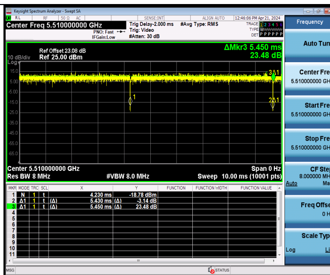
11N40MIMO Ant9 5510
