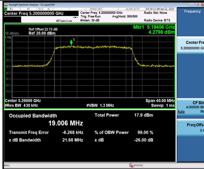
11AX20MIMO Ant9 5200
