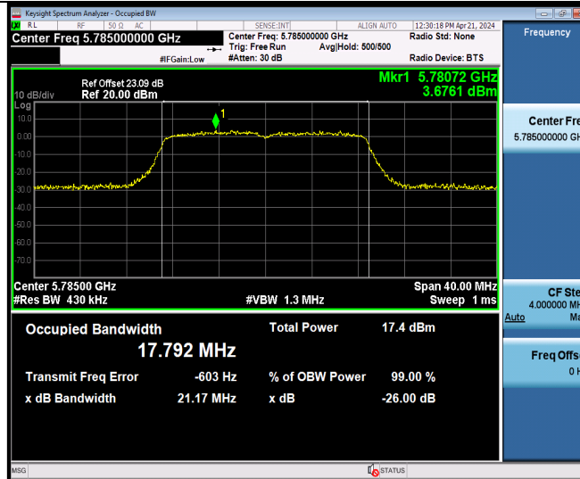
11N20MIMO Ant9 5785
