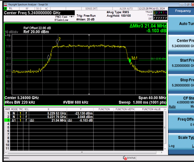
11AX20MIMO Ant9 5240
