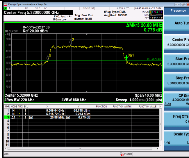
11AX20MIMO Ant9 5320
