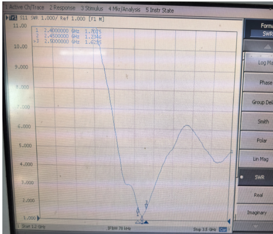
天线驻波比 Antenna SWR
