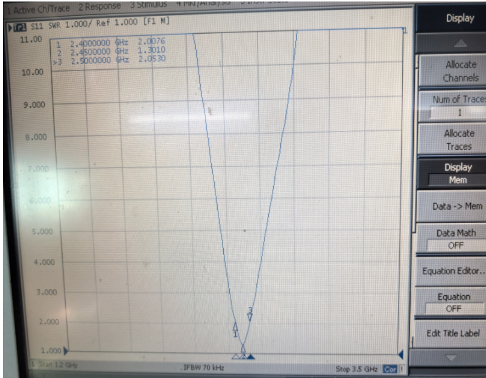
天线驻波比 Antenna SWR
