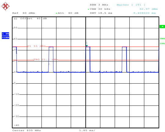
835MHz - GSM
