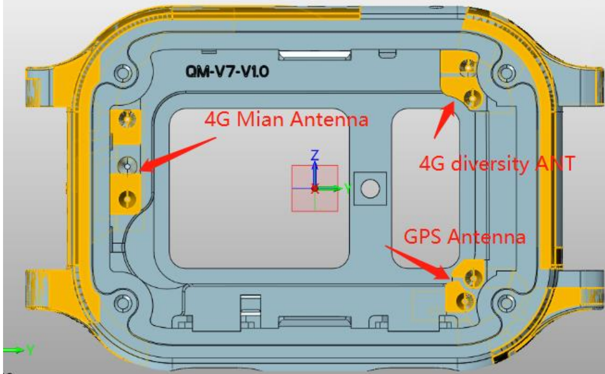
EUT Back
