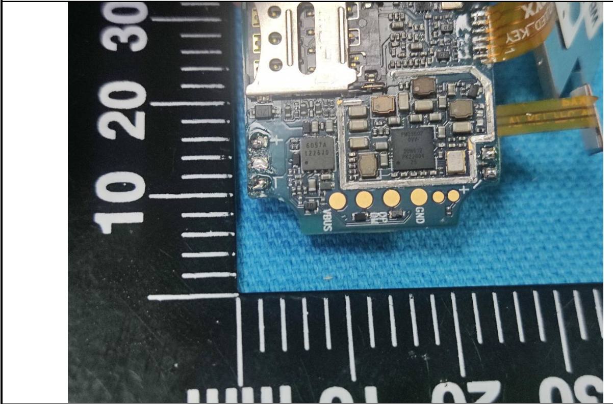
EUT Photo
