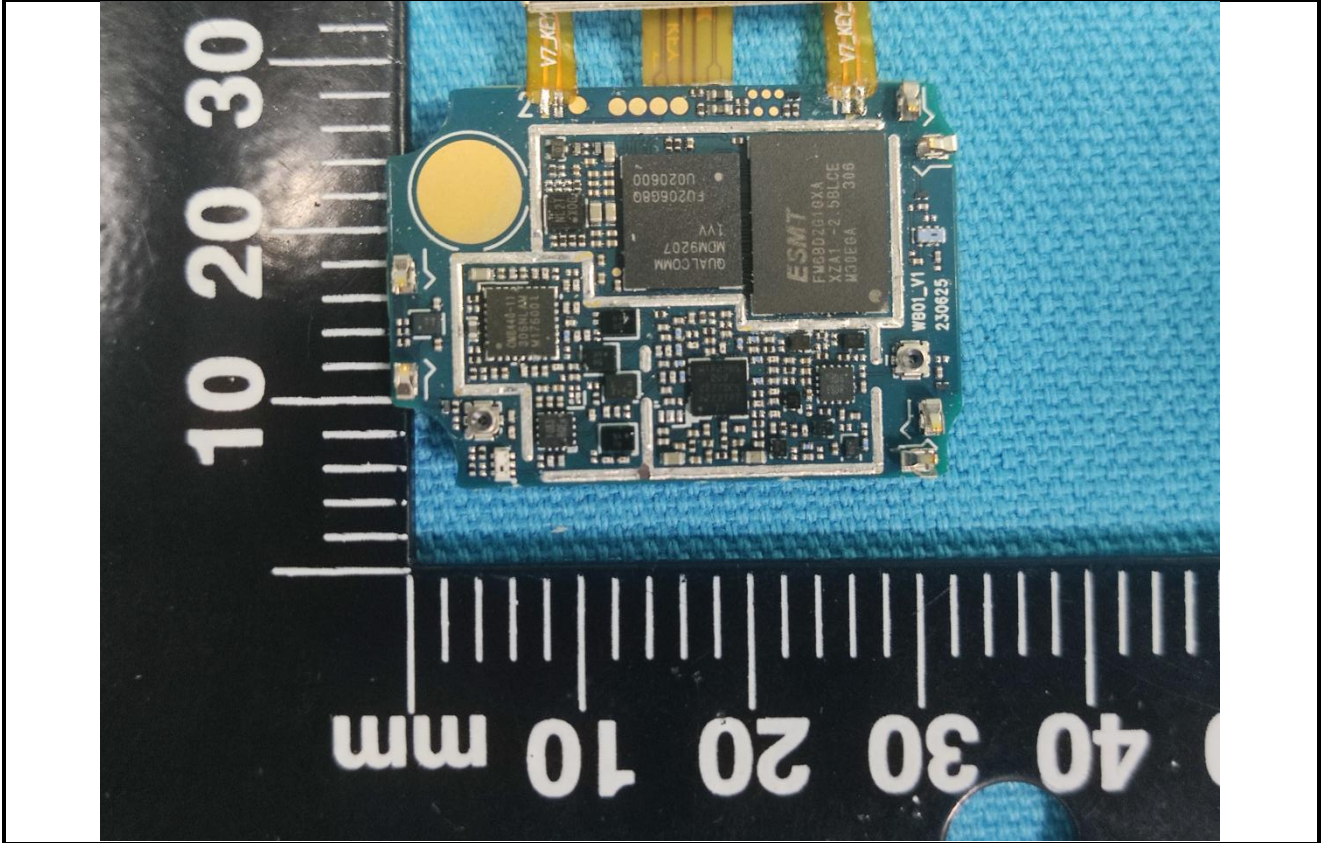
EUT Photo
