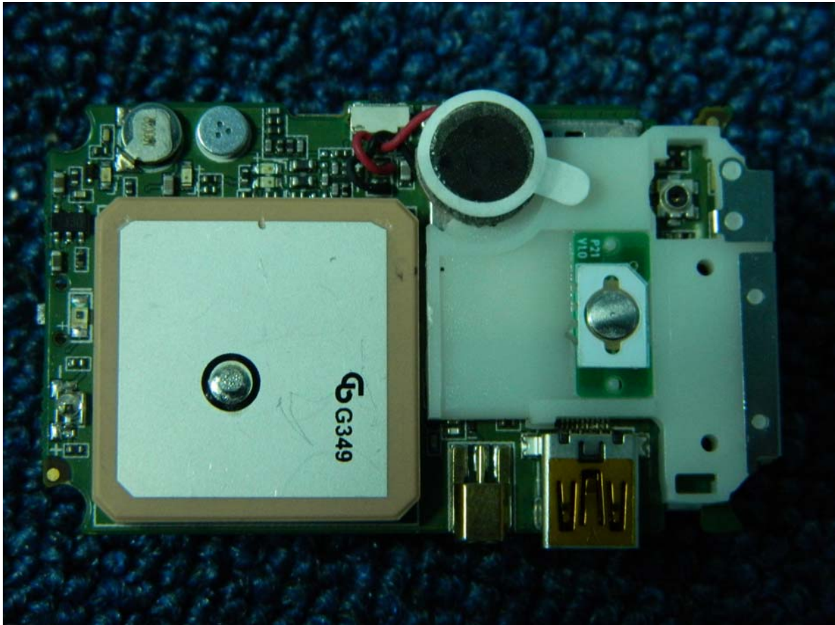
Fig. 1 PCBA (obverse)
