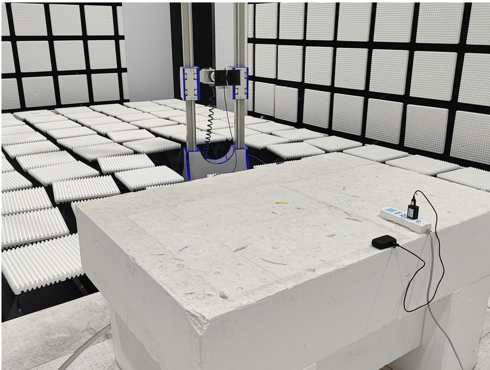
RE_1GHz-18GHz
