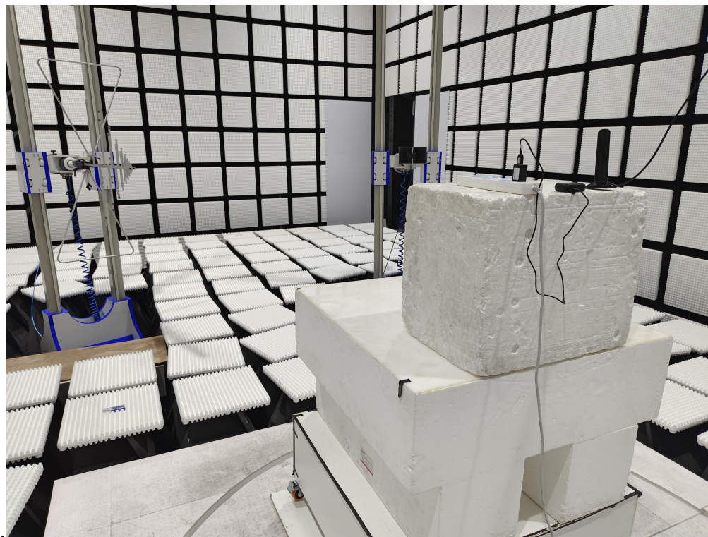
RSE_1GHz-18GHz
