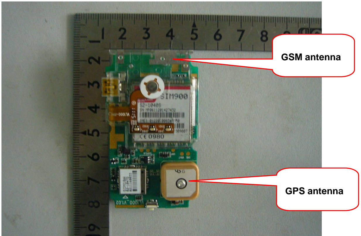
Top View-01
