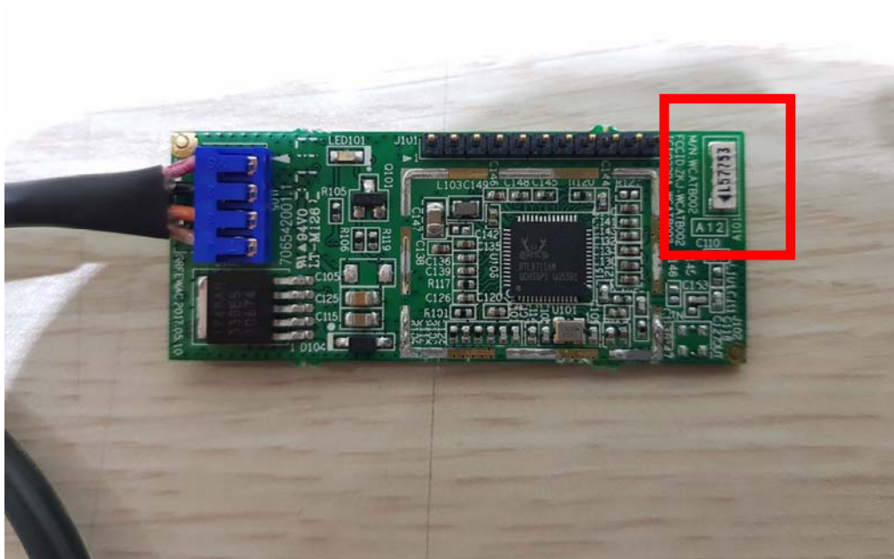
Antenna
